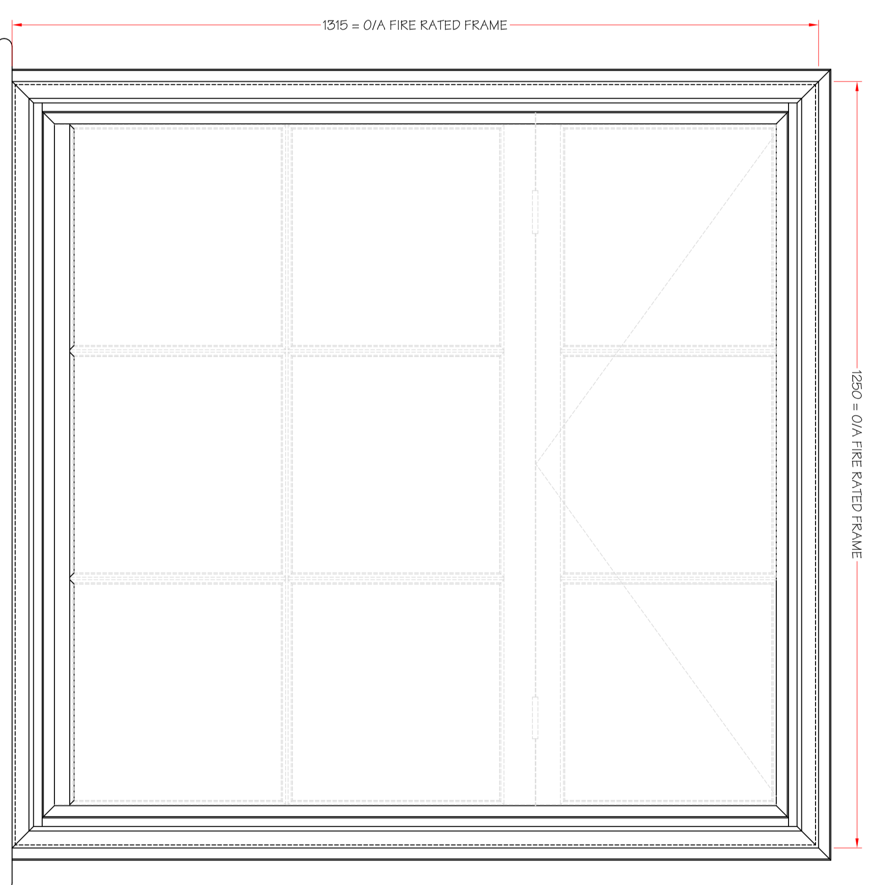
N.T.S. INTERNAL ELEVATION
